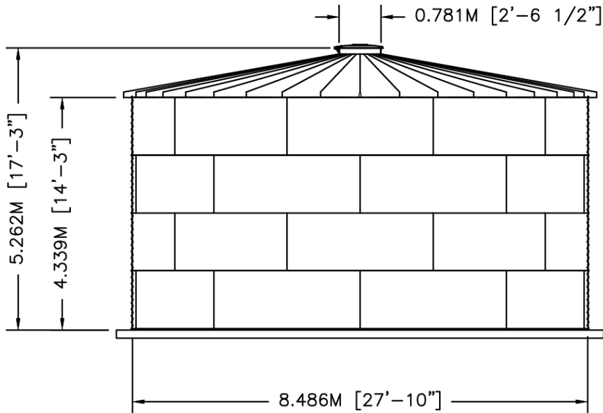
ELEVATION
